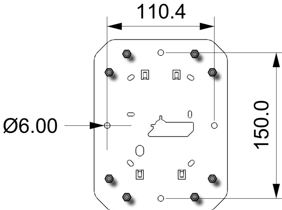
Bakstycke med fästhål för extra bultar
