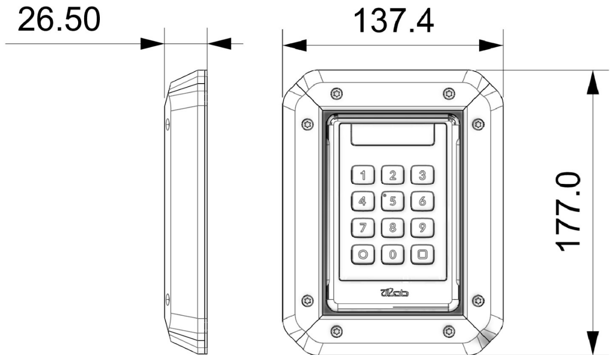
Måttsättning komplett enhet
